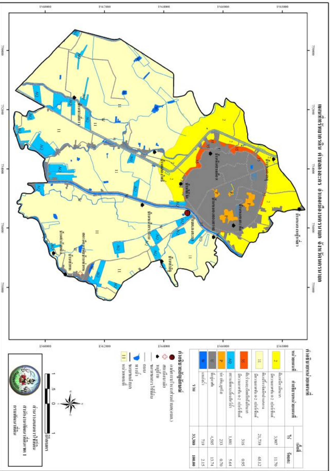
รูปที่ 3-1 แผนที่ทรัพยากรดิน ตำบลดงละคร อำเภอเมืองจันทบุรี จังหวัดจันทบุรี
